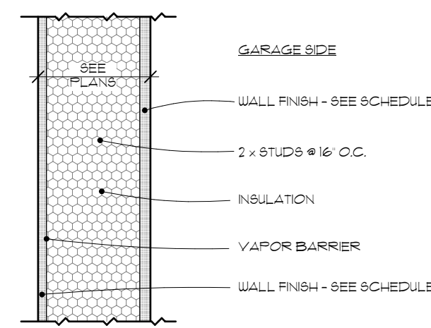
WALL TYPE C SCALE: 1/2" = 1'-0"
