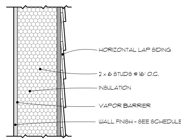
WALL TYPE A SCALE: 1/2" = 1'-0"
