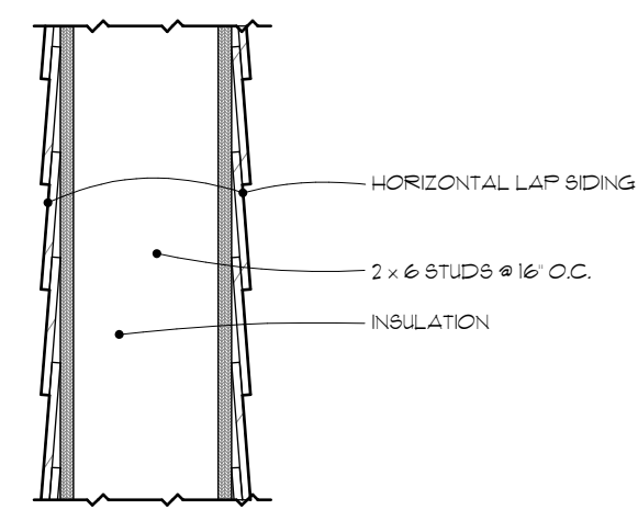
WALL TYPE D SCALE: 1/2" = 1'-0"
