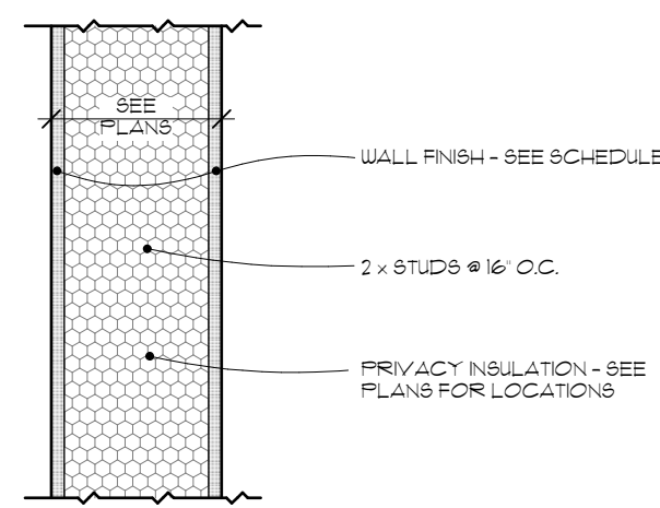
WALL TYPE B SCALE: 1/2" = 1'-0"
